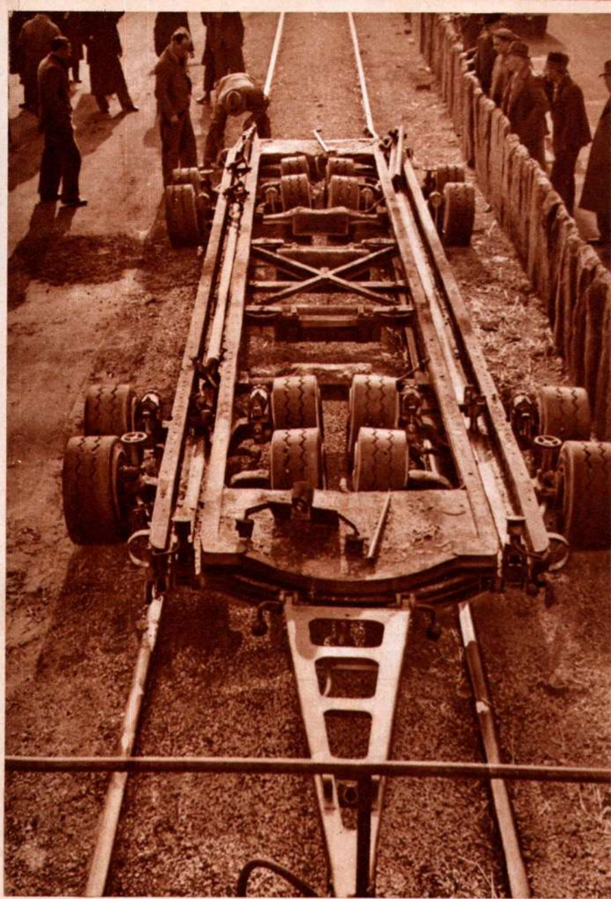
Sopra: Il carrello trasportatore, munito di ben 16 ruote. Di fianco: la potente trattrice a motore Diesel di 100 HP. Sotto: Il convoglio in salita. Noteremo ancora che la velocità di corsa varia dai 5 ai 15 km. orari e che possono essere superate salite a carico pieno sino a pendenza dell'8,7 %.
