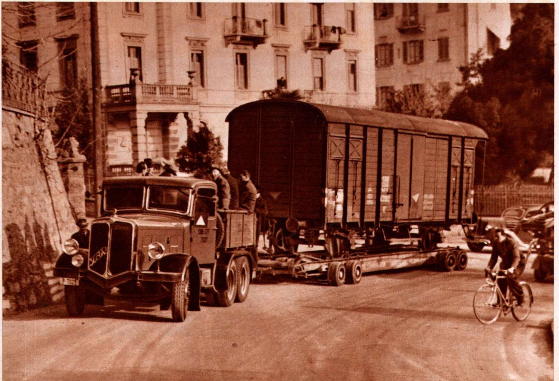
Sopra: Il carrello trasportatore, munito di ben 16 ruote. Di fianco: la potente trattrice a motore Diesel di 100 HP. Sotto: Il convoglio in salita. Noteremo ancora che la velocità di corsa varia dai 5 ai 15 km. orari e che possono essere superate salite a carico pieno sino a pendenza dell'8,7 %.
